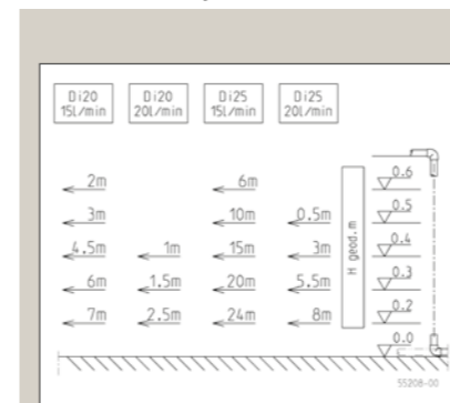
Höhen-/Weitendiagramm
