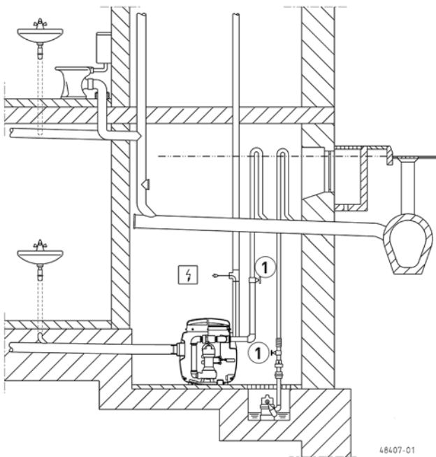
Einbaubeispiel Hebefix 200
