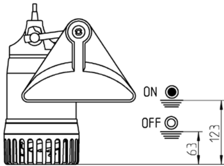
Dimensions flotteur spécial UV3 S (mm)
