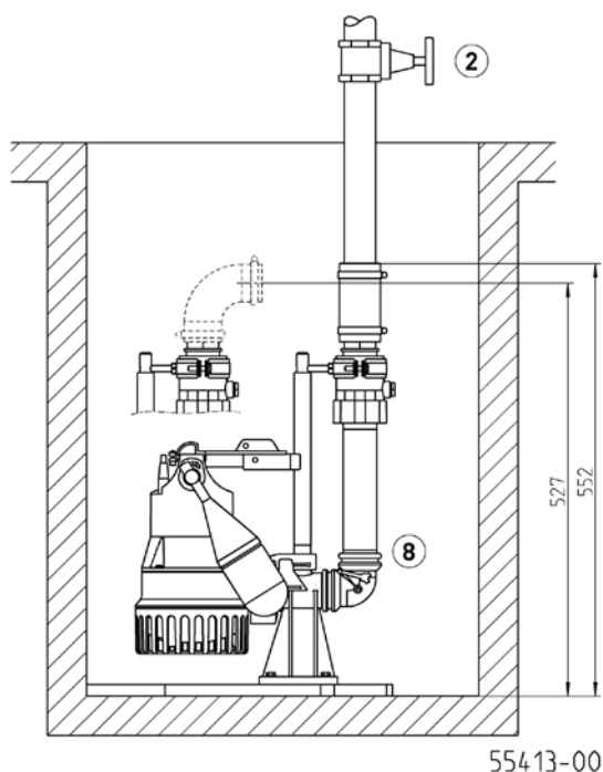
Przykład zabudowy i wymiary główne Easyfix 32 Single (mm)
