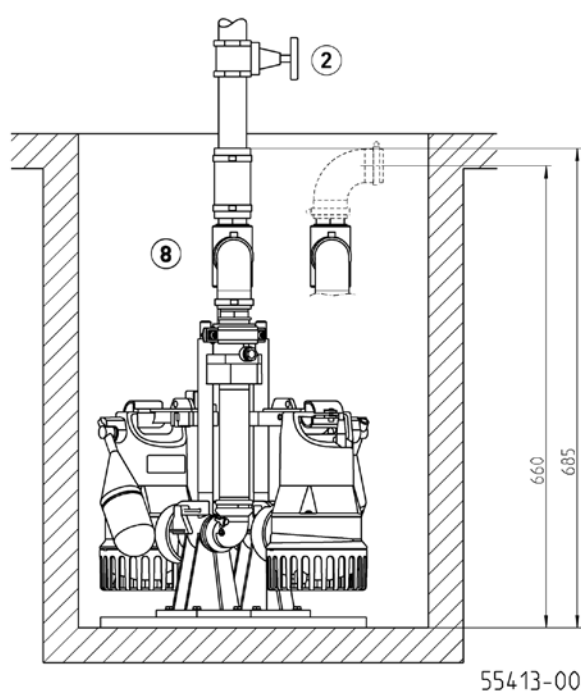
Przykład zabudowy i wymiary główne Easyfix 32 Duo (mm)
