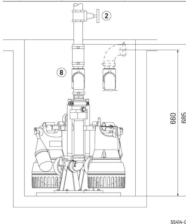
Exemple de montage et dimensions Easyfix 32 Duo (mm)
