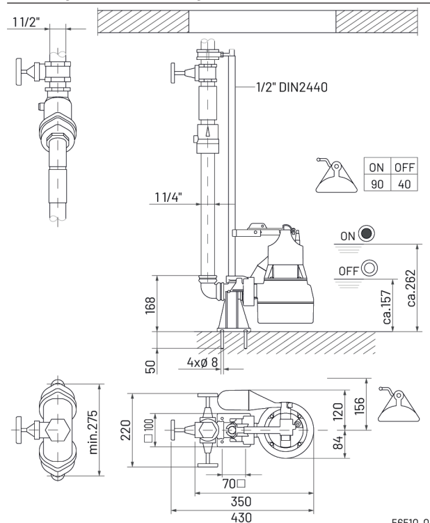
Afmetingen en schakelhoogtes GR 32 (mm)
