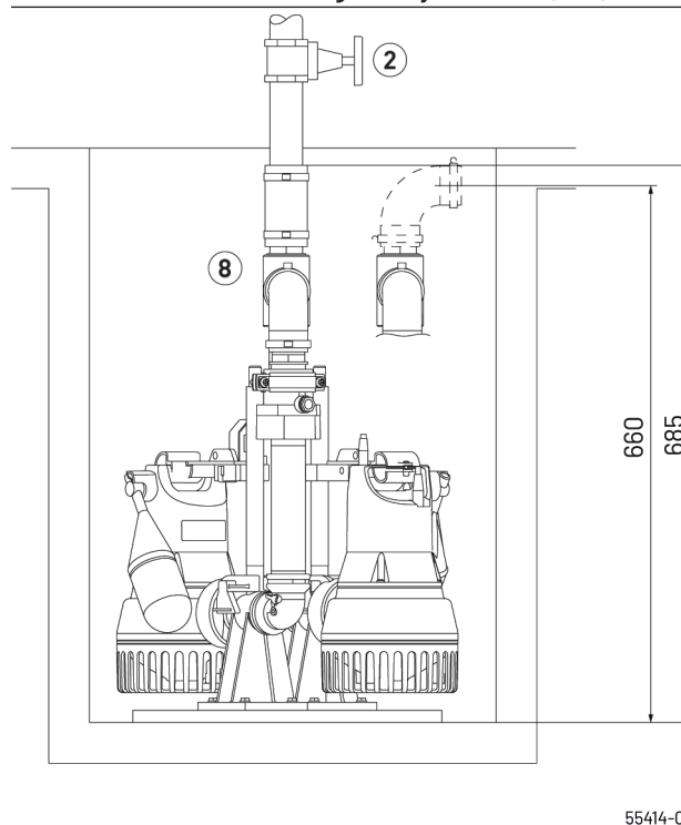
Inbouwvoorbeeld en afmetingen Easyfix 32 Duo (mm)
