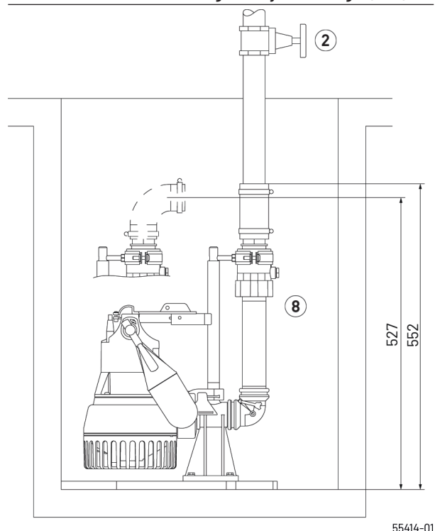
Inbouwvoorbeeld en afmetingen Easyfix 32 Single (mm)
