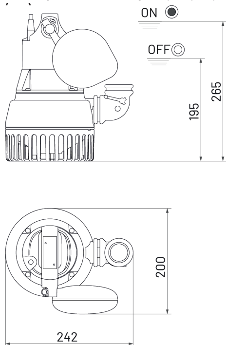
Afmetingen en schakelhoogtes spec. pompvlotter
