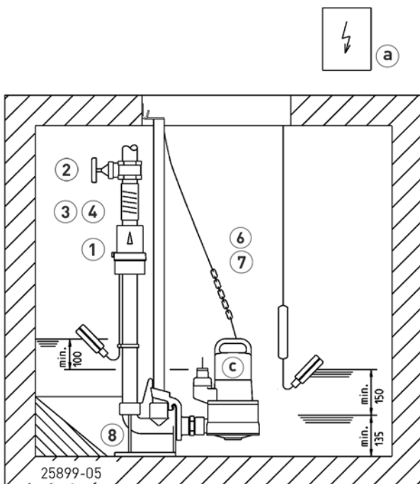
Exemple de montage poste simple (GR)
